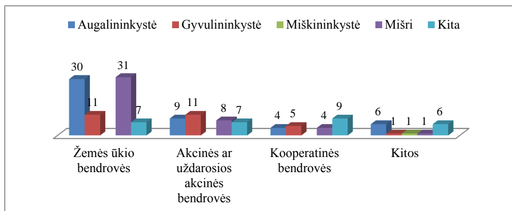
2 pav. Pagal teisinę formą suskirstytų įmonių pagrindinė veikla
