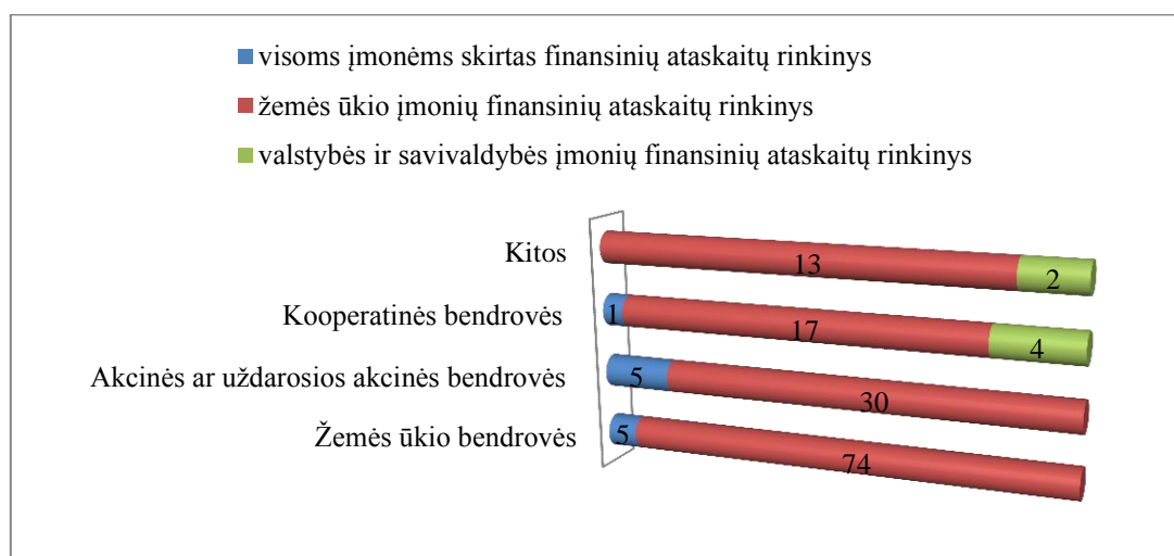
3 pav. Finansinių ataskaitų rinkinių pasirinkimas pagal įmonių teisinę formą
