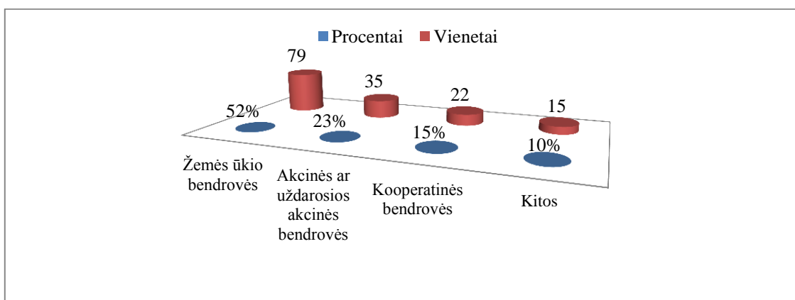
1 pav. Įmonių, atsakiusių į klausimyną, pasiskirstymas pagal teisinę formą
