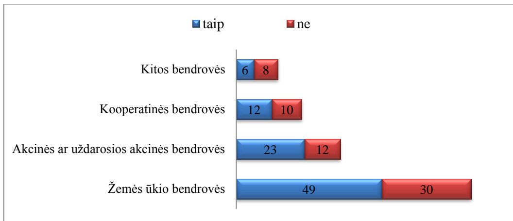
5 pav. Įmonių nuomonė dėl žemės ūkio įmonių pelno (nuostolių) ataskaitos formos panaikinimo
