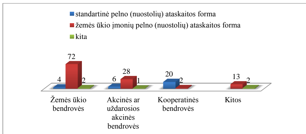
4 pav. Pelno (nuostolių) ataskaitos formos, kurias rinkosi įmonės, rengusios žemės ūkio įmonės finansinių ataskaitų rinkinį
